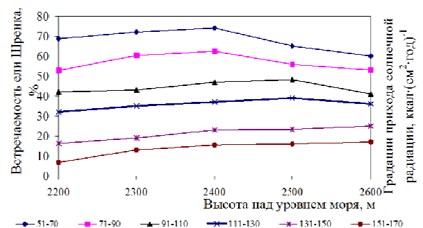
Рисунок 1 – Графическая модель возможной встречаемости ели Шренка в зависимости от инсоляции склона и абсолютной высоты местности для Иссык-Кульского лесхоза
